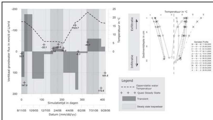
Figuur 5: Tijdsafhankelijke simulatie de flux van punt 7 in de periode 11-08-2005 tot 28-09-2006. Aan de linkerzijde van de grafiek worden de berekende grondwater fluxen tussen 11.08.2005 en 28.09.2006 getoond. De kruisjes staan voor Quasi-steady state resultaten, de donkergrijze rechthoeken duiden de gemiddelde flux tussen twee metingen aan. Het diagram aan de rechterkant toont de gemeten temperatuurprofielen die voor de analyse gebruikt worden.
